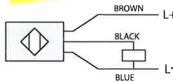
Diagram 2 PNP Cable
